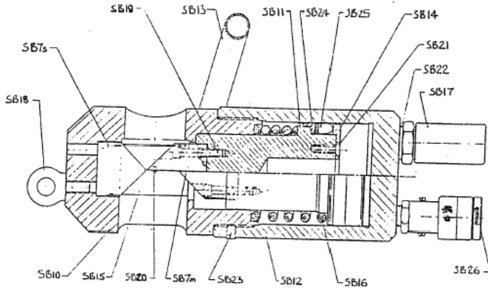
SIMM SB1 25mm 螺栓切割器剖面配件示意图
